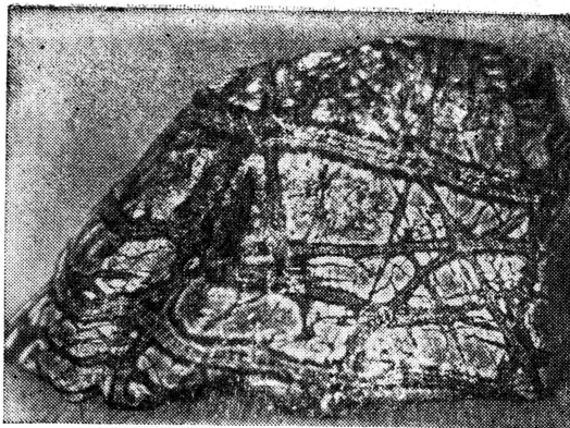
Каменный цветок — арагонит. Седонское месторождение на Кавказе.
