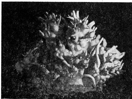
Окаменевшее древнее животное михелиния. 300 миллионов лет.
