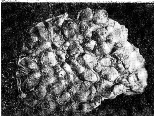
Ракушечник. Найден в Туркменской ССР, кишлак Кель-Ата.
